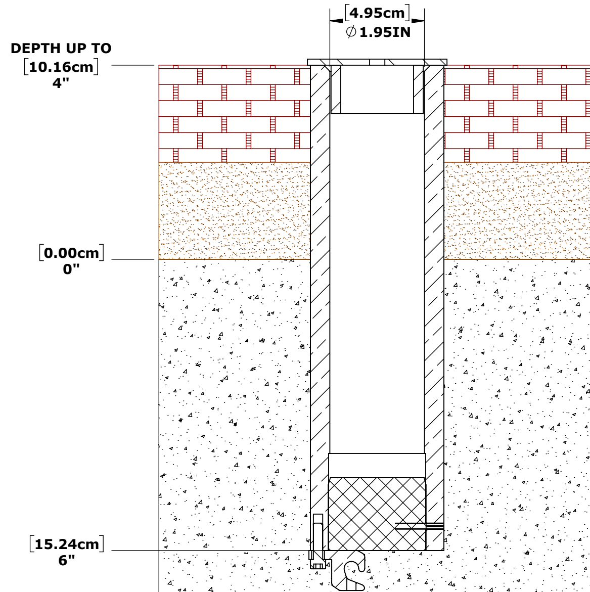
SECTION A-A SCALE 1 : 2
